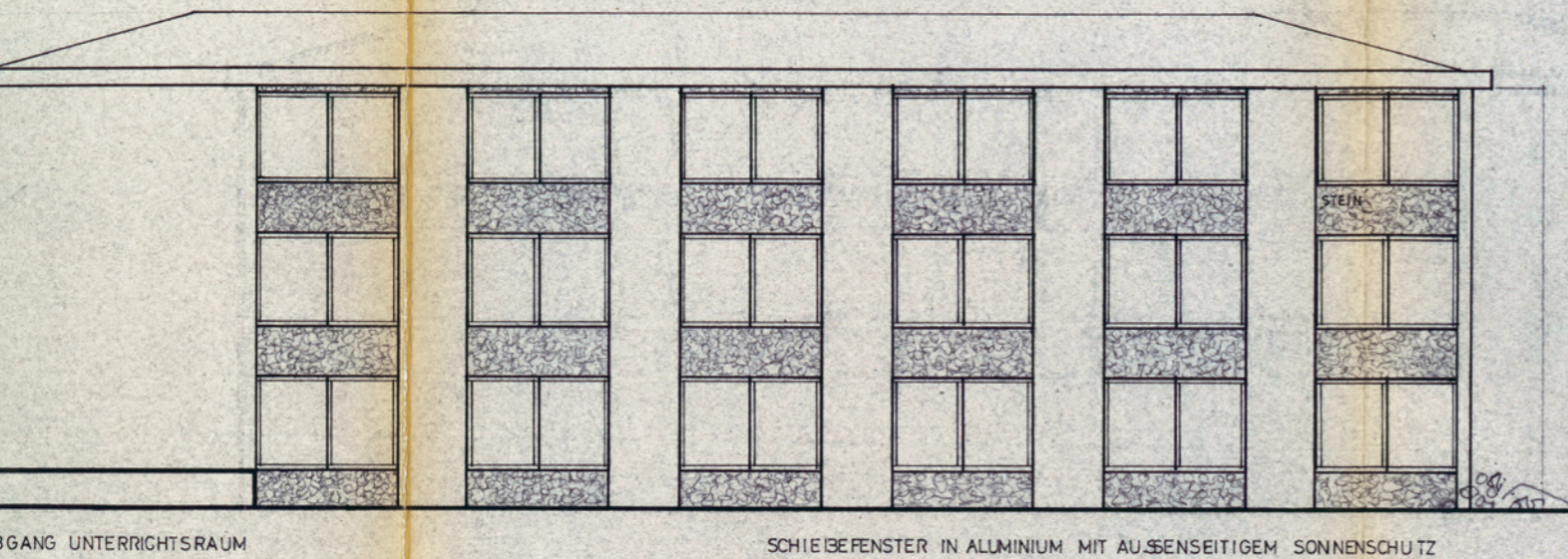
Außenansicht nach Planzeichnungen vom Juni 1963: oben Eingangsseite zur Poststraße, unten Büfensterfront zur Ringpromenade
